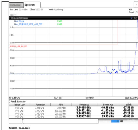
Band2(3450-3550)-10MHz-QPSK-43040-50RB#0-PASS
