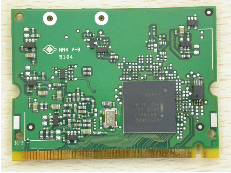
RF Module
