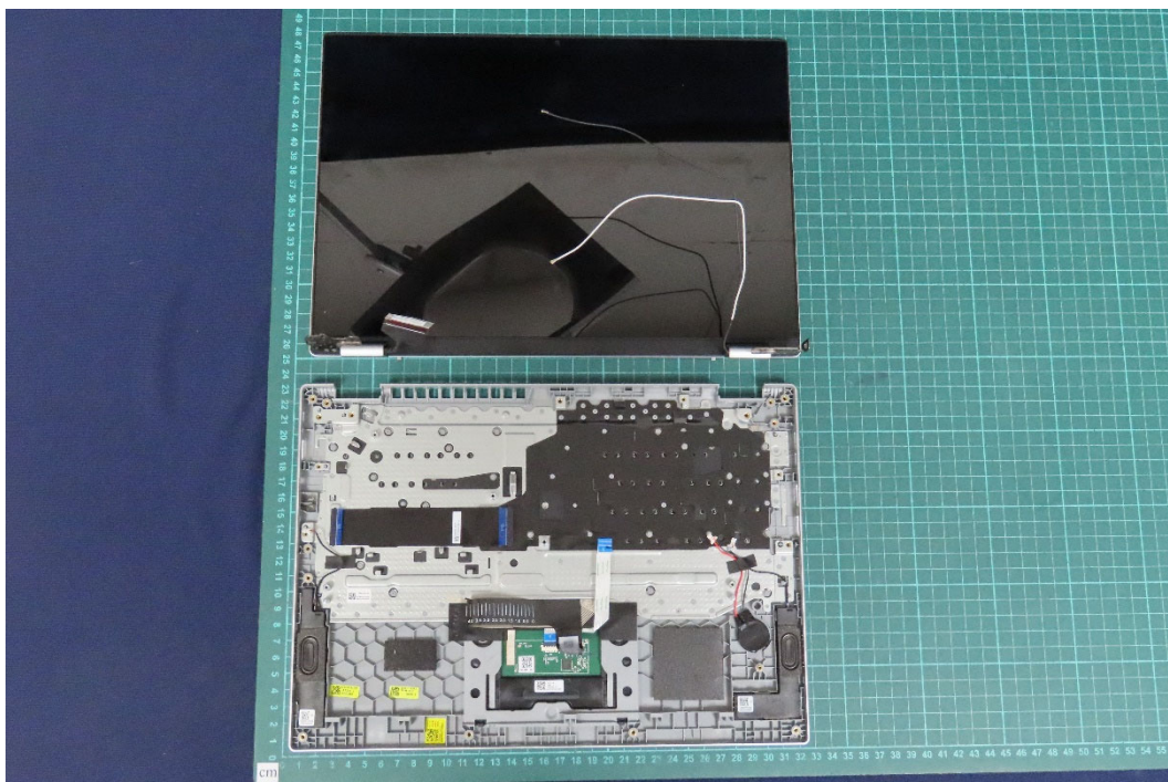
(36) EUT Photo
