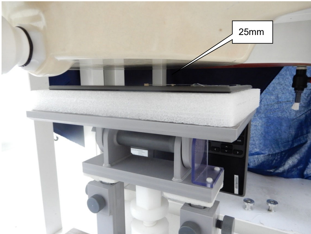
EUT Back(NB)
