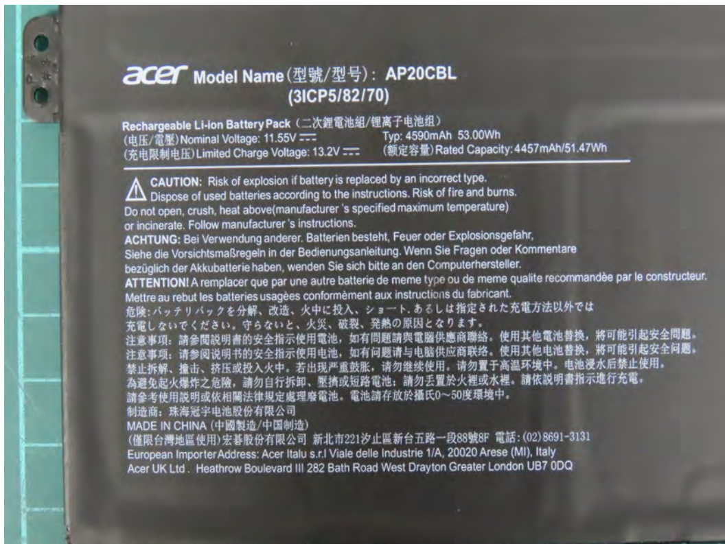
(18) EUT Photo
