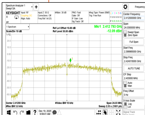
802.11ax_20MHz_Chain0_2412MHz_RU242
