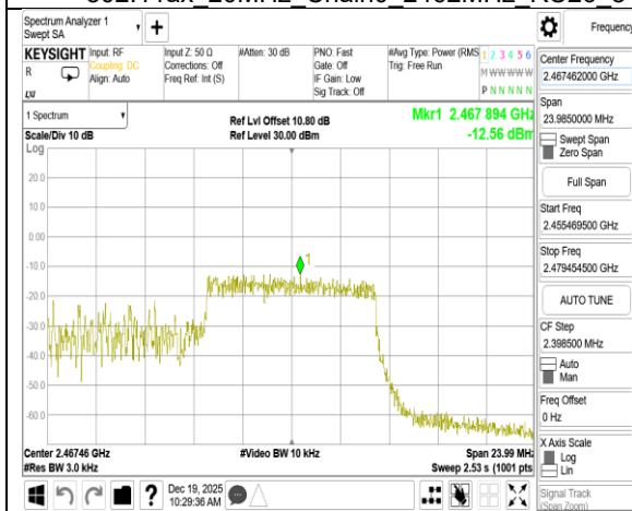
802.11ax 20MHz Chain0 2462MHz RU106 54
