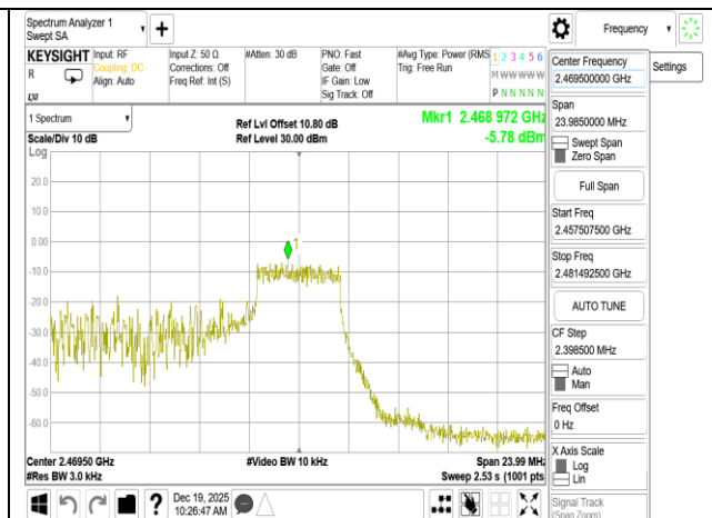
802.11ax 20MHz Chain0 2462MHz RU52 40
