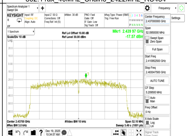
802.11ax 40MHz Chain0 2437MHz RU484
