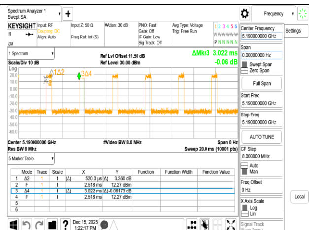
802.11ax_40MHz_Chain0_5190MHz
