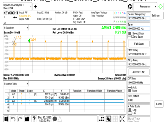
802.11ax 80MHz Chain0 5210MHz RU996
