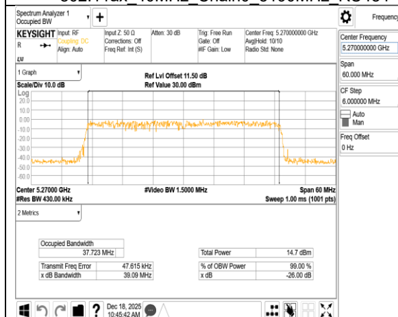
802.11ax 40MHz Chain0 5270MHz RU484
