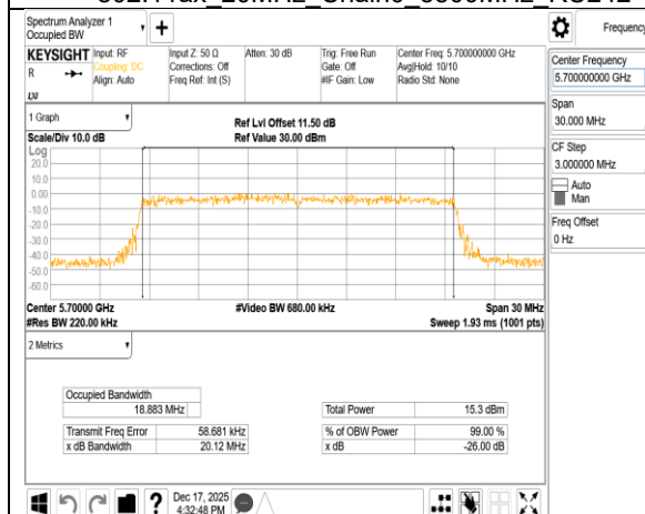
802.11ax 20MHz Chain0 5700MHz RU242
