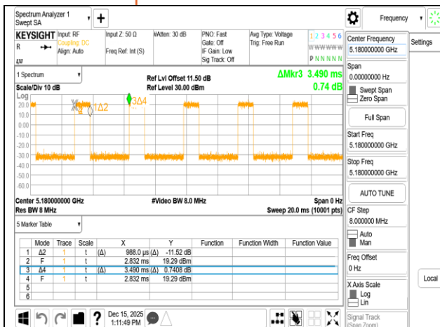
802.11ax_20MHz_Chain0_5180MHz
