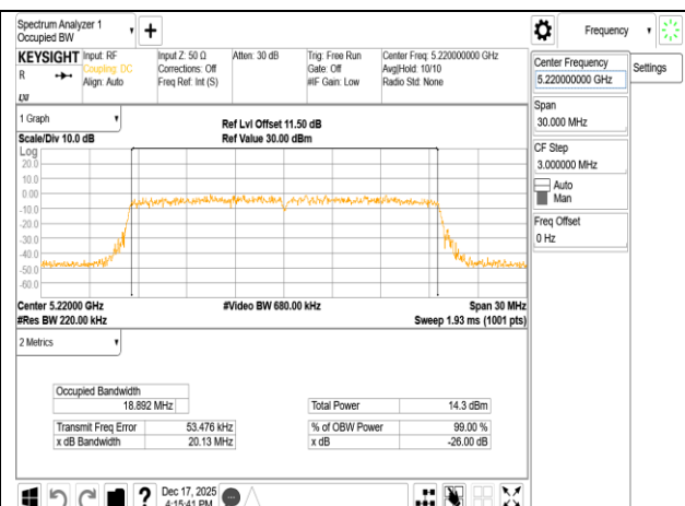
802.11ax 20MHz Chain0 5220MHz RU242
