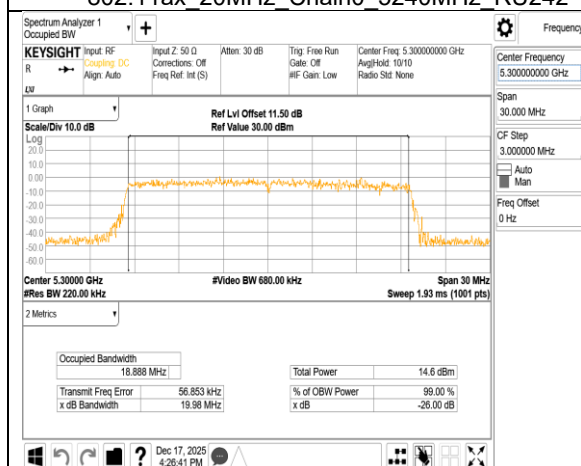
802.11ax 20MHz Chain0 5300MHz RU242
