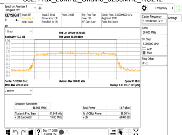
802.11ax 20MHz Chain0 5320MHz RU242
