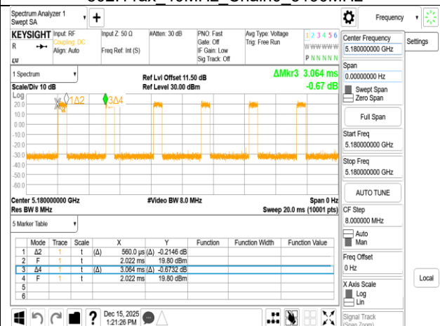
802.11ax_20MHz_Chain0_5180MHz RU242
