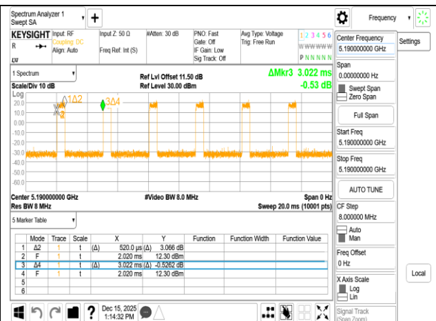
802.11ax_40MHz_Chain0_5190MHz
