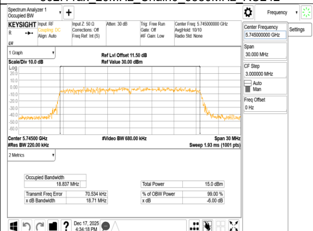
802.11ax 20MHz Chain0 5745MHz RU242
