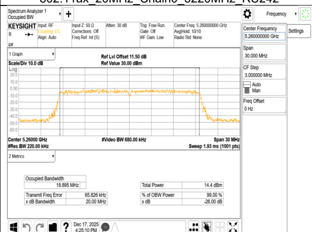
802.11ax 20MHz Chain0 5260MHz RU242
