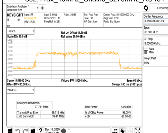
802.11ax 40MHz Chain0 5510MHz RU484
