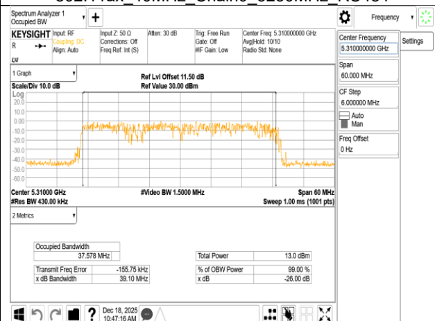
802.11ax 40MHz Chain0 5310MHz RU484
