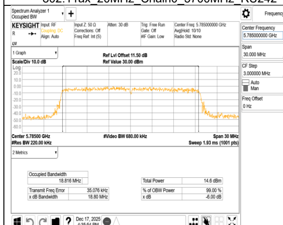
802.11ax 20MHz Chain0 5785MHz RU242
