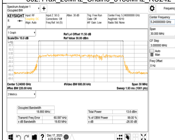
802.11ax 20MHz Chain0 5240MHz RU242
