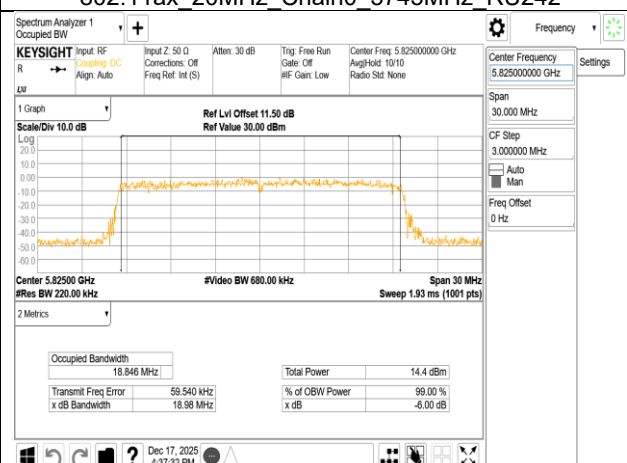
802.11ax 20MHz Chain0 5825MHz RU242
