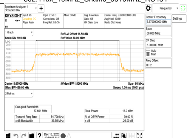
802.11ax 40MHz Chain0 5670MHz RU484
