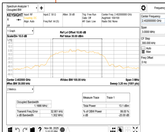
OBW 20dB 8DPSK 3M DH5 2402MHz
