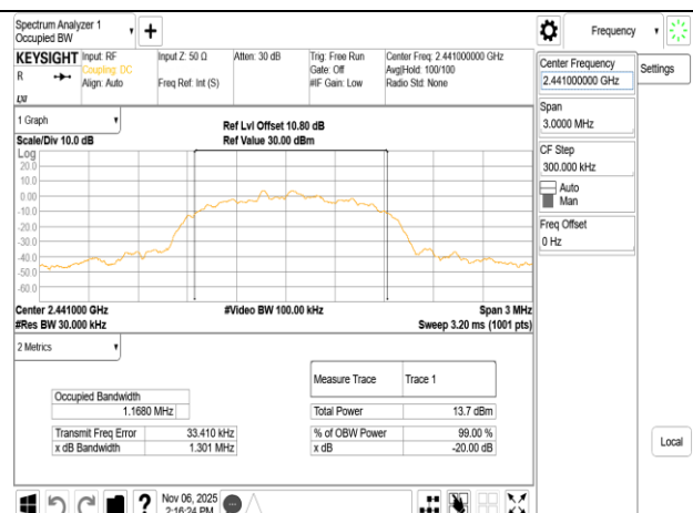
OBW 20dB 8DPSK 3M DH5 2441MHz
