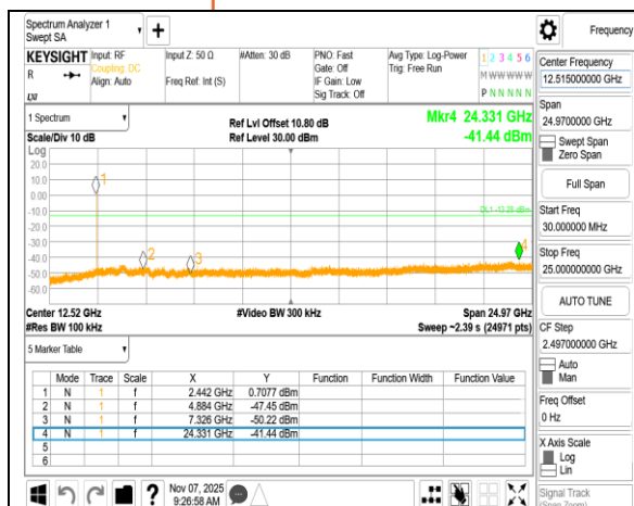
Spurious Emission BLE 2M MidCH20-2442MHz
