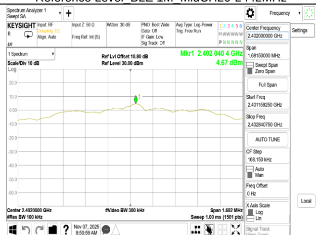
Reference Level BLE 2M LowCH00-2402MHz
