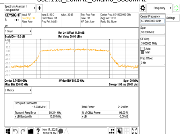
802.11a 20MHz Chain0 5745MHz
