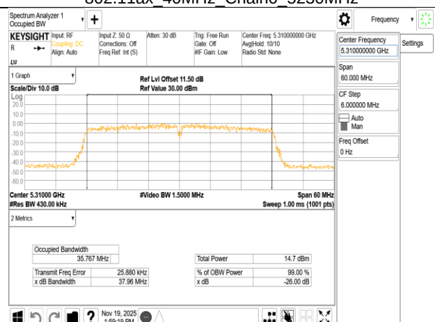
802.11ax 40MHz Chain0 5310MHz
