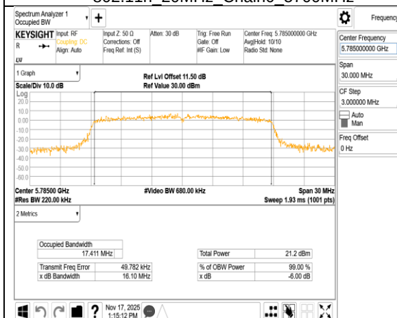
802.11n 20MHz Chain0 5785MHz
