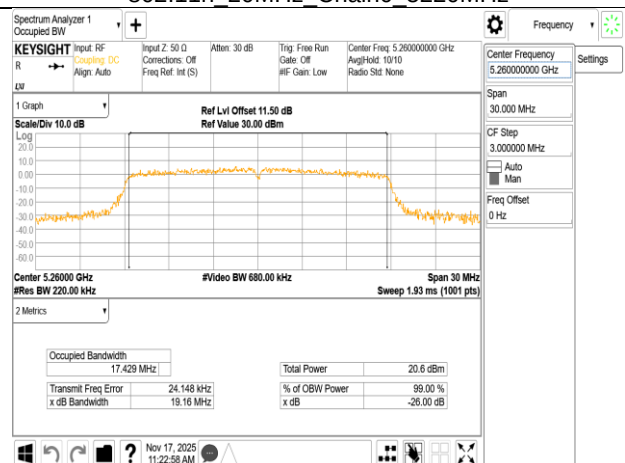
802.11n 20MHz Chain0 5260MHz
