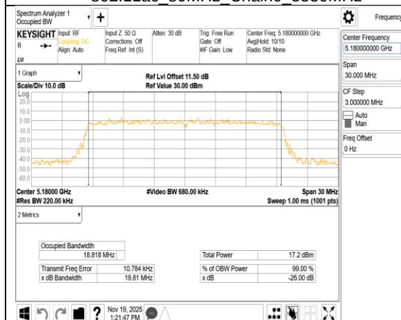
802.11ax 20MHz Chain0 5180MHz
