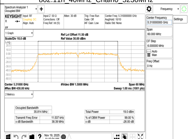
802.11n 40MHz Chain0 5310MHz
