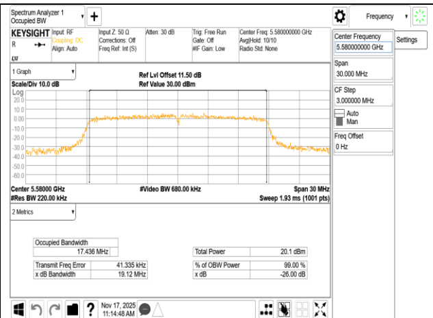
802.11n 20MHz Chain0 5580MHz
