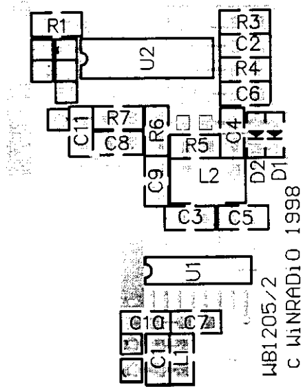
DIGITAL BFO - TOP
