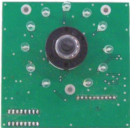
BSW3 Bottom Side
