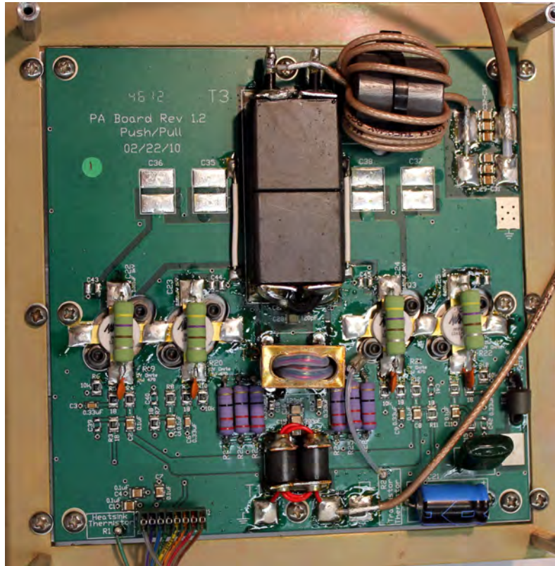
PAM-606 (PA module) bottom
