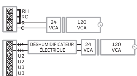
RACCORDEMENT TYPE D'UN DÉSHUMIDIFICATEUR ÉLECTRIQUE (DÉSHUMIDIFICATEUR POUR TOUTE LA MAISON)
