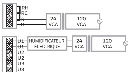
RACCORDEMENT TYPE D'UN HUMIDIFICATEUR ÉLECTRIQUE
