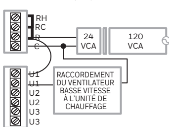
RACCORDEMENT TYPE D'UN VENTILATEUR À VITESSE VARIABLE POUR LA DÉSHUMIDIFICATION EN BASSE VITESSE (ANY)
