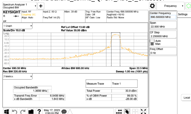
Cat-M1 Band71_15MHz_QPSK_RB6_0_CH133397
