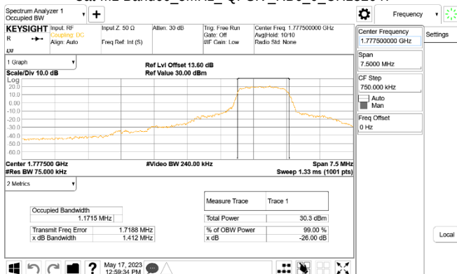
Cat-M1 Band66_5MHz_QPSK_RB6_0_CH132647
