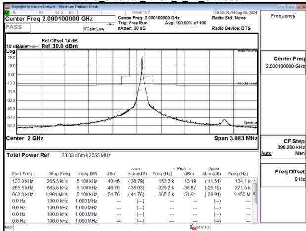
Band23 3.75kHz BPSK 1_47_CH25600
