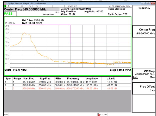
Band Edge_Band26_15MHz_PUSCH_841.5MHz_Chain0
