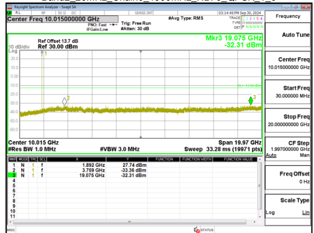
Band2_20MHz_Chain0_1900MHz_NBI 0_QPSK_1_0
