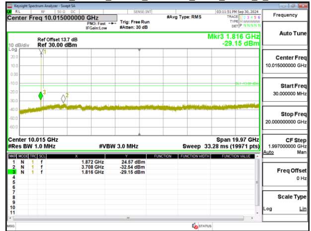
Band2_20MHz_Chain0_1900MHz_NBI 0_QPSK_1_0
