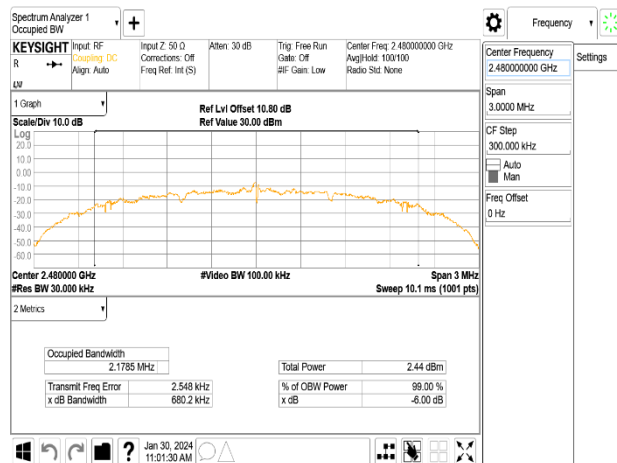
IC OBW_Zigbee_HighCH26-2480MHz
