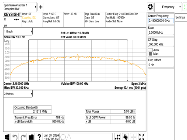
IC OBW_Zigbee_HighCH26-2480MHz
