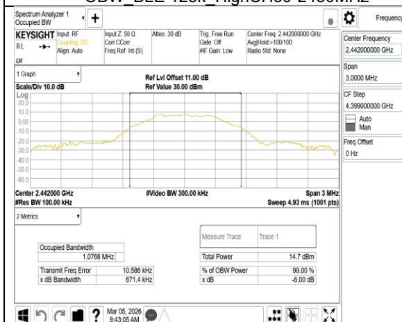
OBW_BLE 500k_MidCH20-2442MHz
