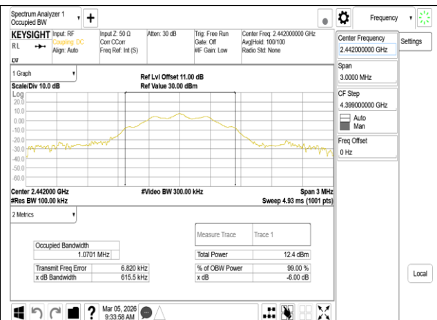
OBW_BLE 125k_MidCH20-2442MHz
