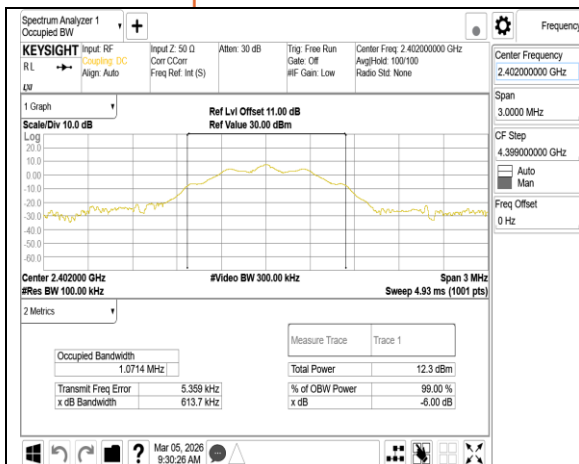
OBW_BLE 125k_LowCH00-2402MHz
