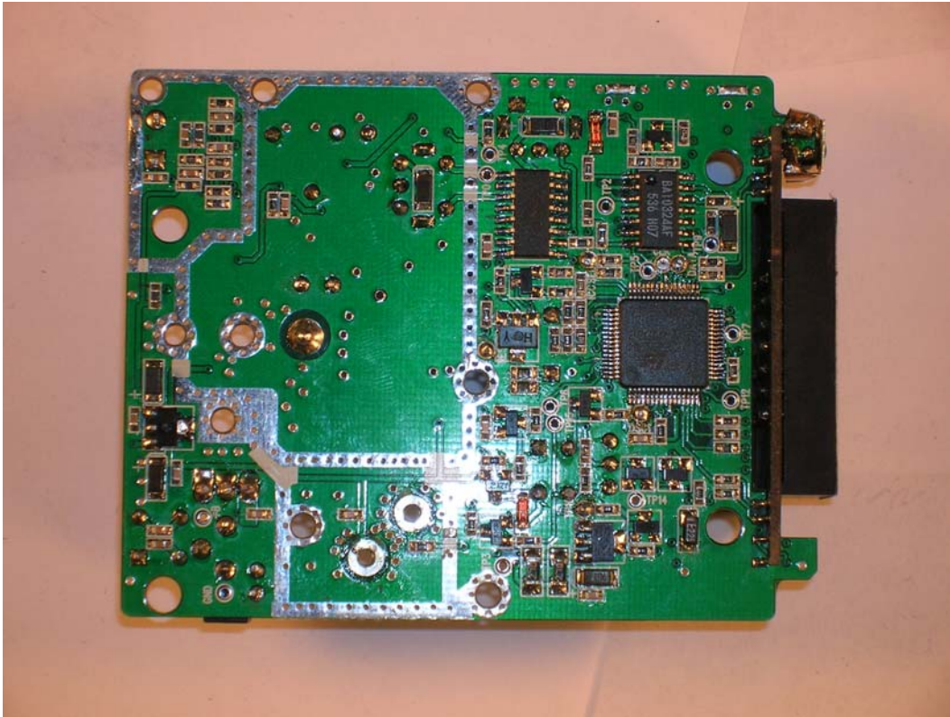
XTR 220 PCB bottom
