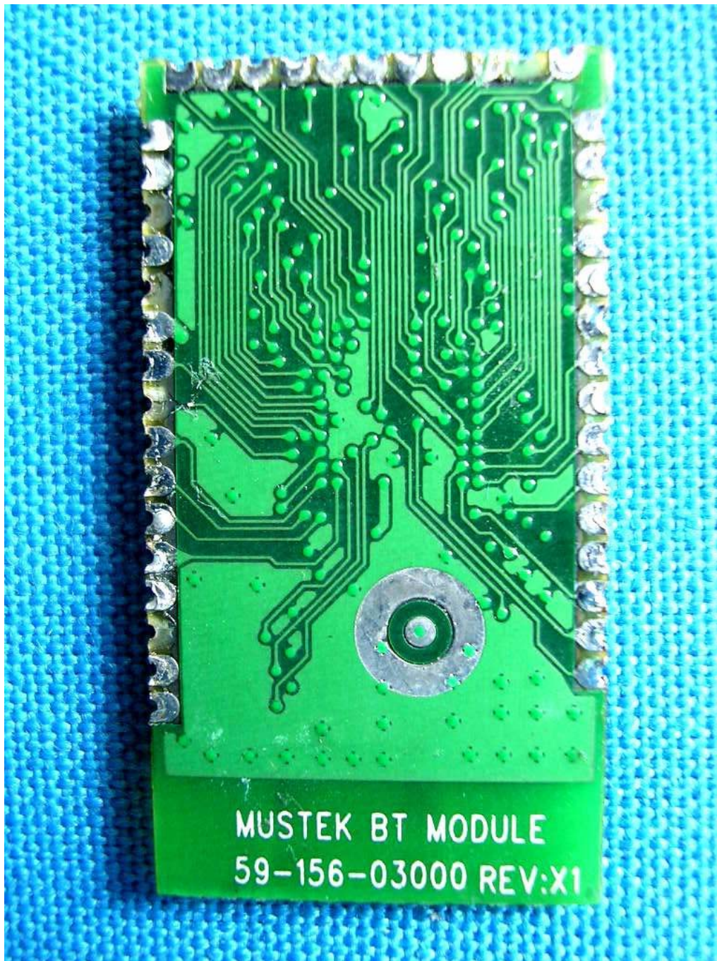
(10) EUT Photo
