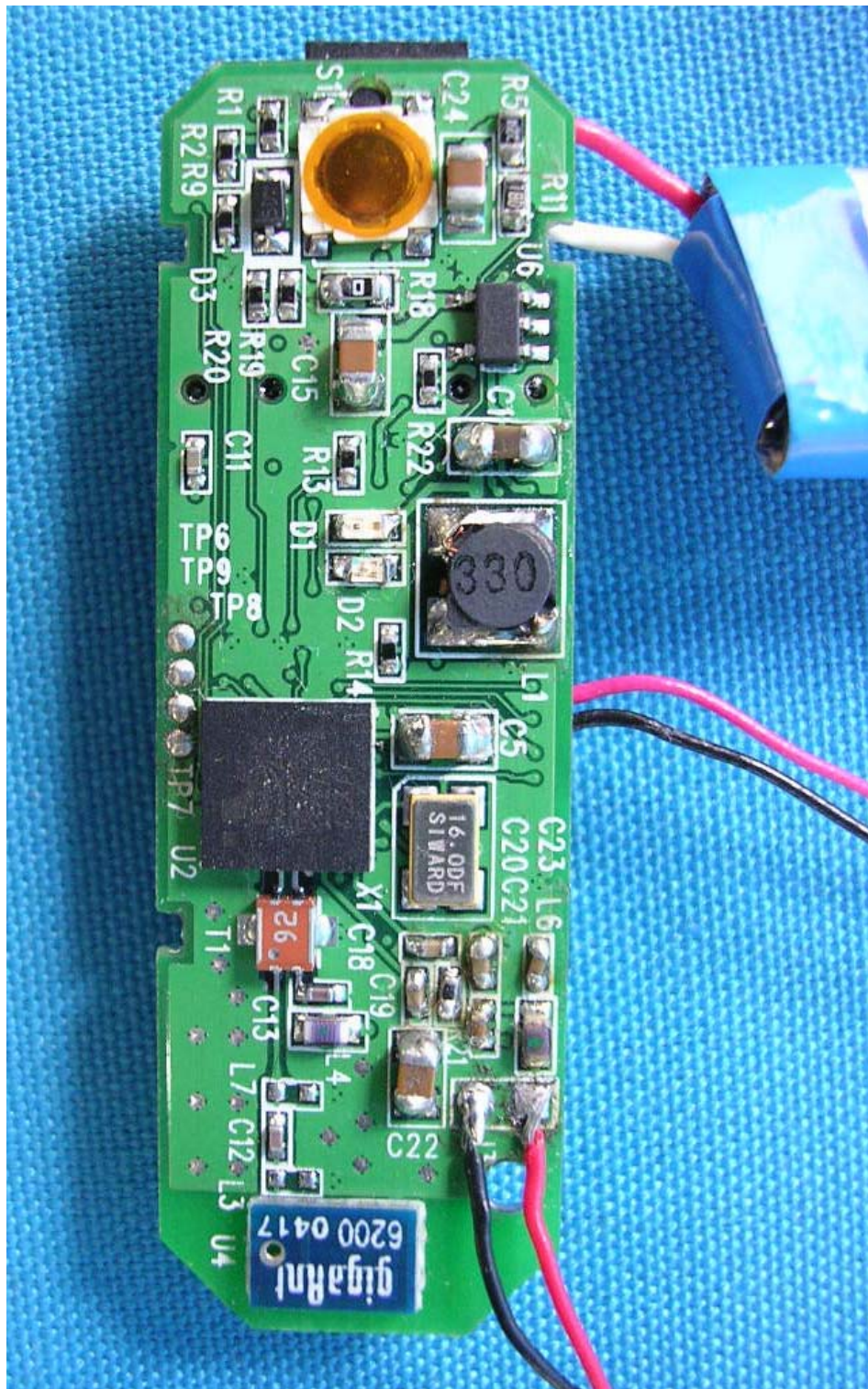
(4) EUT Photo
