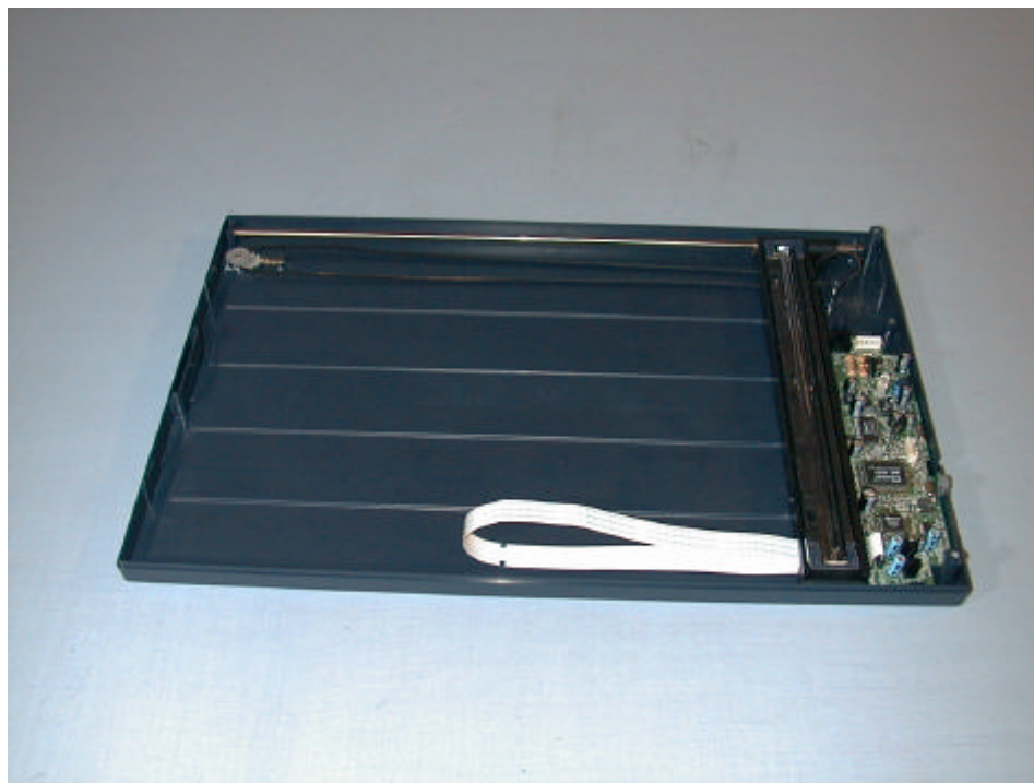
(10)EUT Photo
