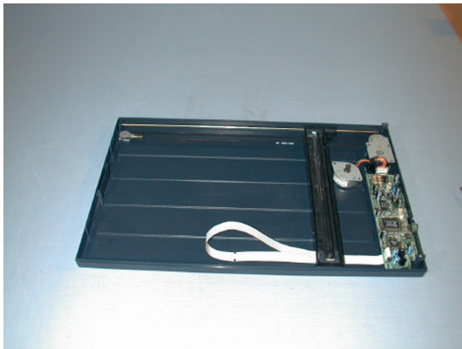
(6)EUT Photo
