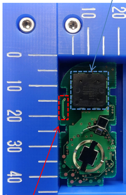
Antenna (Tx)
