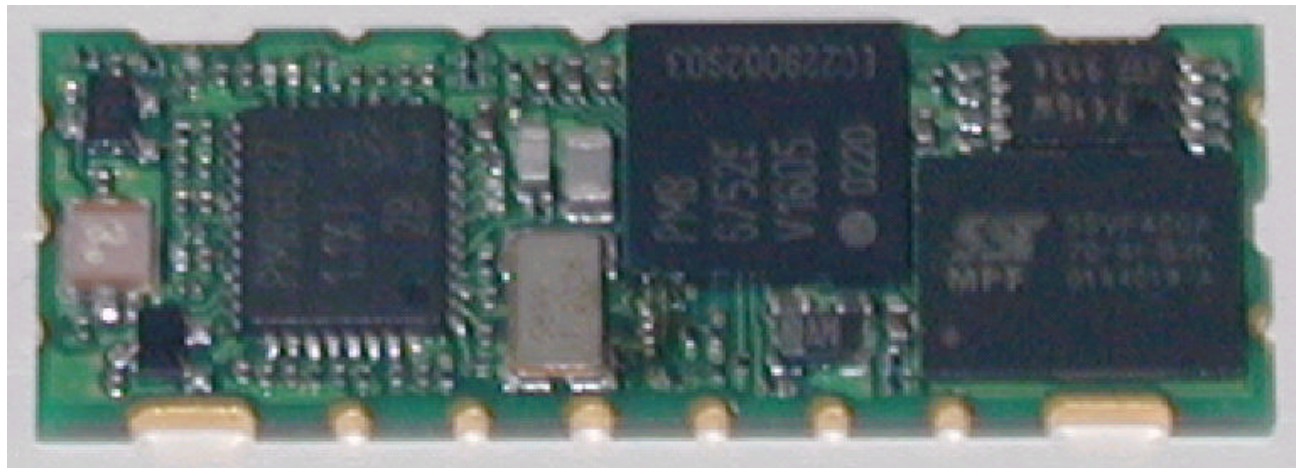
Bluetooth module IC (Component side)
