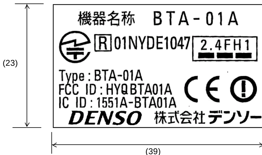
Fig. 4.5.3. Label Layout
