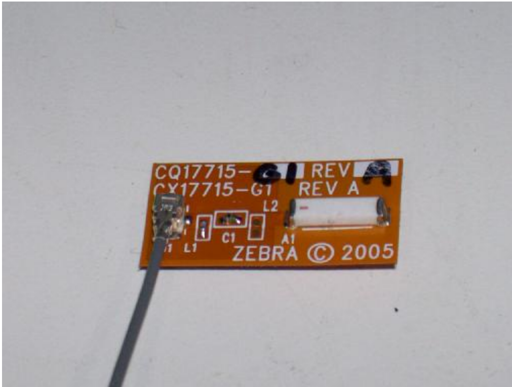
Photo 1: CQ17715-G1 Antenna
