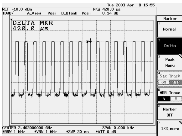
2402MHz
