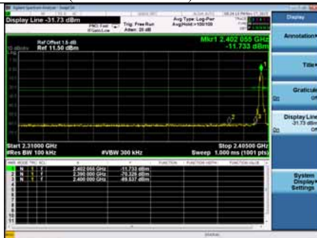
2402MHz(2.3GHz – 2.4GHz)
