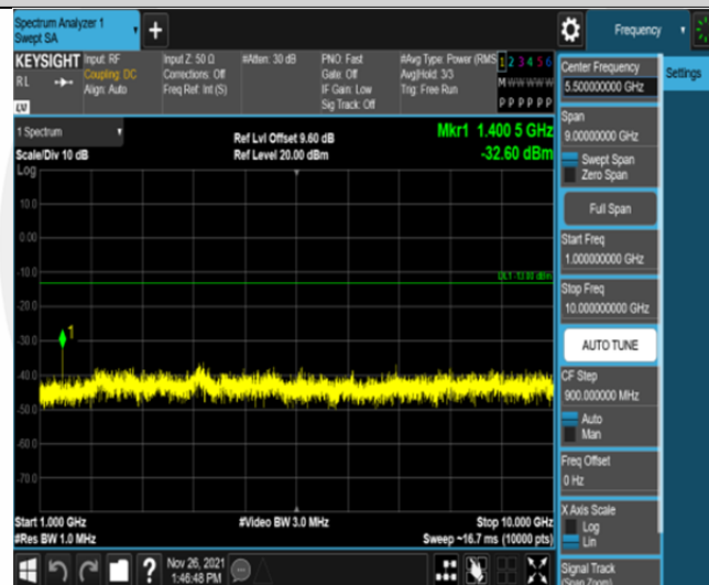
Band12-1.4MHz-QPSK-23017-6RB#0-Range2:1000~10000MHz
