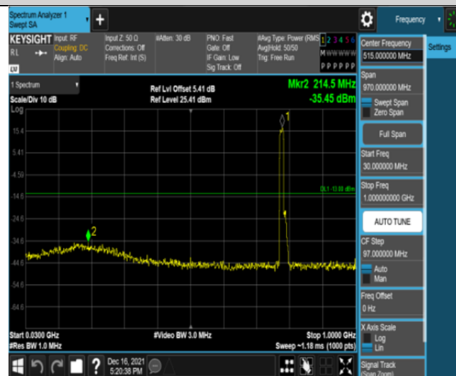
Band13-5MHz-QPSK-23230-25RB#0-Range1:30~1000MHz
