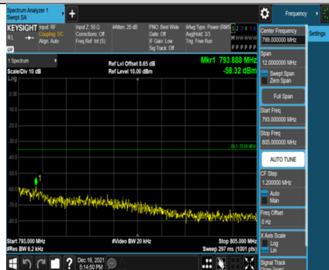
Band13-5MHz-QPSK-23205-25RB#0-Range4:793~805MHz
