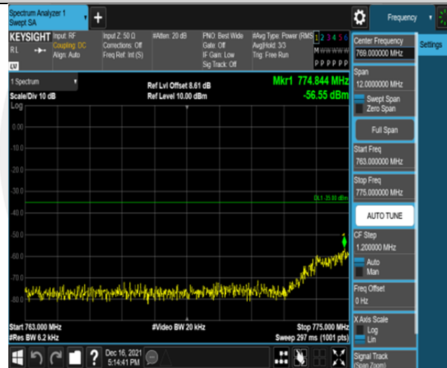
Band13-5MHz-QPSK-23205-25RB#0-Range3:763~775MHz
