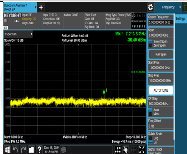
Band13-5MHz-QPSK-23255-25RB#0-Range2:1000~10000MHz
