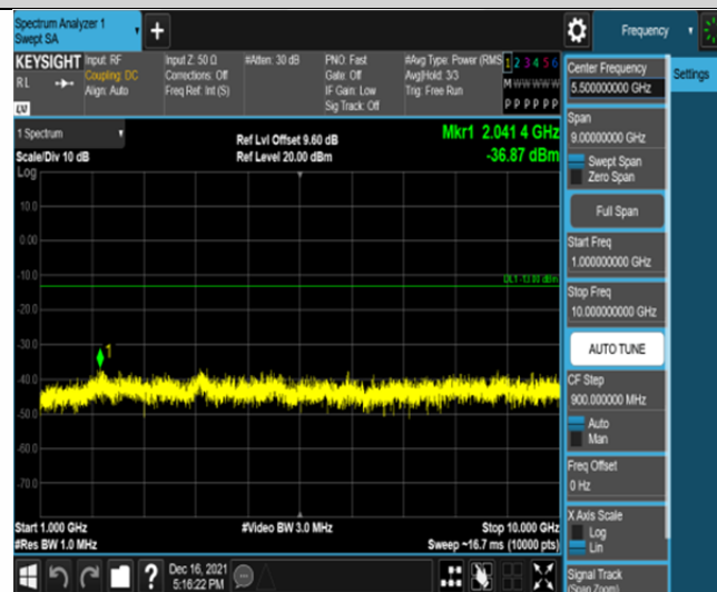
Band13-5MHz-QPSK-23230-25RB#0-Range2:1000~10000MHz
