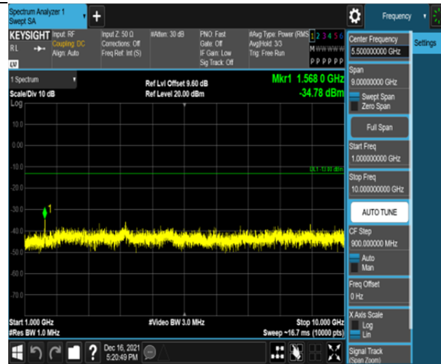
Band13-10MHz-QPSK-23230-50RB#0-Range2:1000~10000MHz
