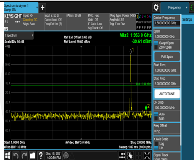
Band2-3MHz-16QAM-18615-15RB#0-Range2:1000~2000MHz
