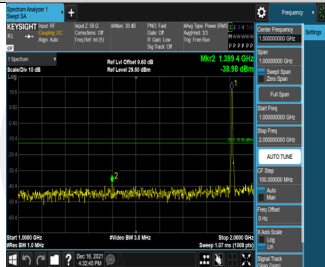
Band2-3MHz-QPSK-19185-15RB#0-Range2:1000~2000MHz
