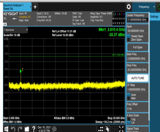
Band2-3MHz-QPSK-19185-15RB#0-Range3:2000~20000MHz
