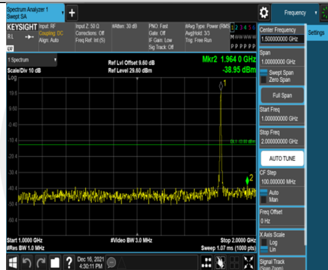
Band2-3MHz-QPSK-18615-15RB#0-Range2:1000~2000MHz
