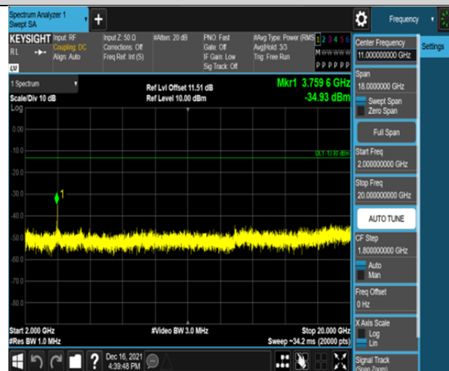
Band2-5MHz-QPSK-18900-25RB#0-Range3:2000~20000MHz
