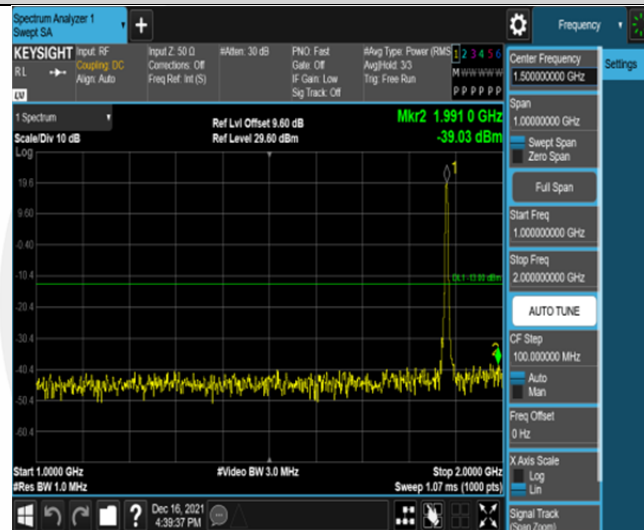
Band2-5MHz-QPSK-18900-25RB#0-Range2:1000~2000MHz
