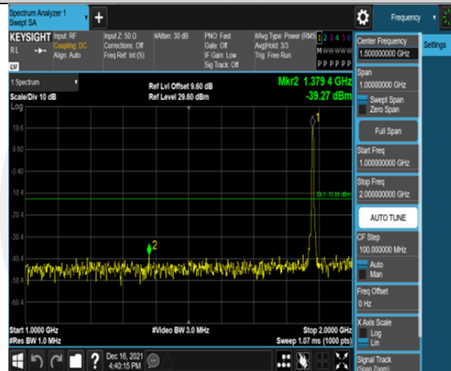
Band2-5MHz-16QAM-18900-25RB#0-Range2:1000~2000MHz
