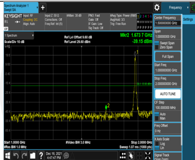
Band2-10MHz-16QAM-18900-50RB#0-Range2:1000~2000MHz
