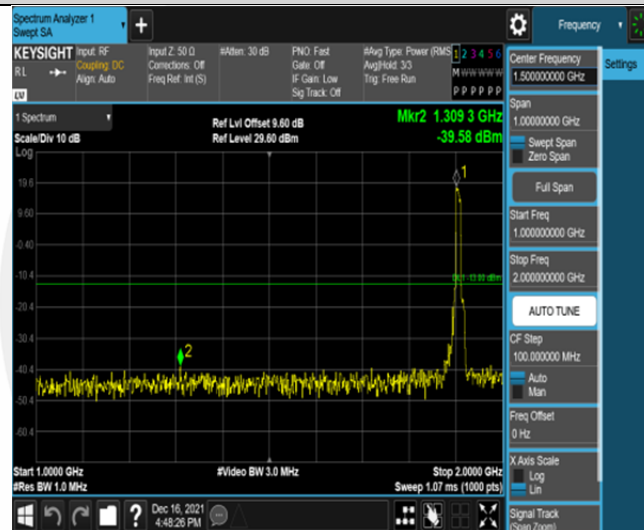
Band2-10MHz-QPSK-19150-50RB#0-Range2:1000~2000MHz
