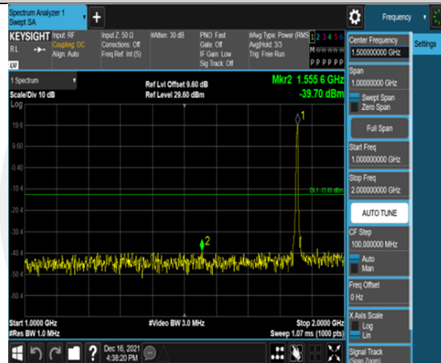
Band2-5MHz-QPSK-18625-25RB#0-Range2:1000~2000MHz
