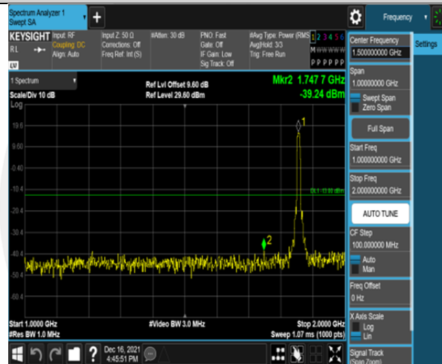
Band2-10MHz-QPSK-18650-50RB#0-Range2:1000~2000MHz
