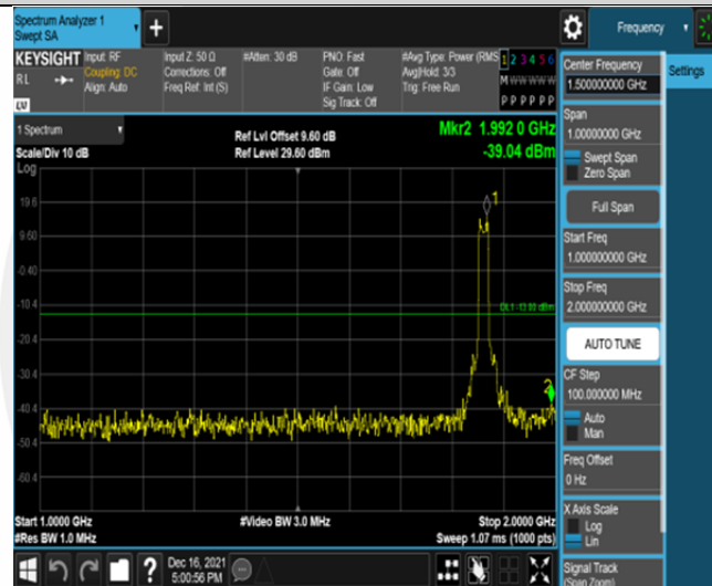
Band2-20MHz-QPSK-18700-100RB#0-Range2:1000~2000MHz
