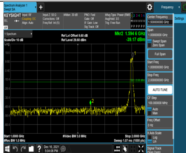
Band2-20MHz-16QAM-19100-100RB#0-Range2:1000~2000MHz
