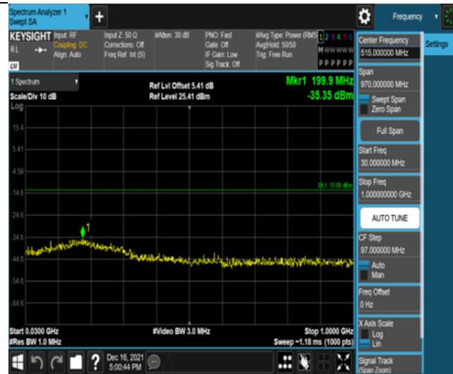
Band2-20MHz-QPSK-18700-100RB#0-Range1:30~1000MHz
