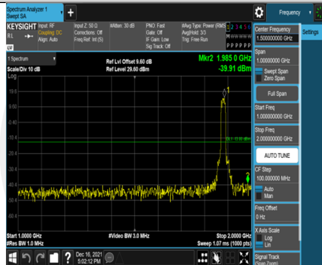
Band2-20MHz-QPSK-18900-100RB#0-Range2:1000~2000MHz
