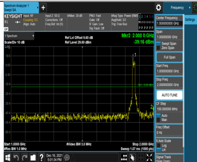
Band2-20MHz-16QAM-18700-100RB#0-Range2:1000~2000MHz
