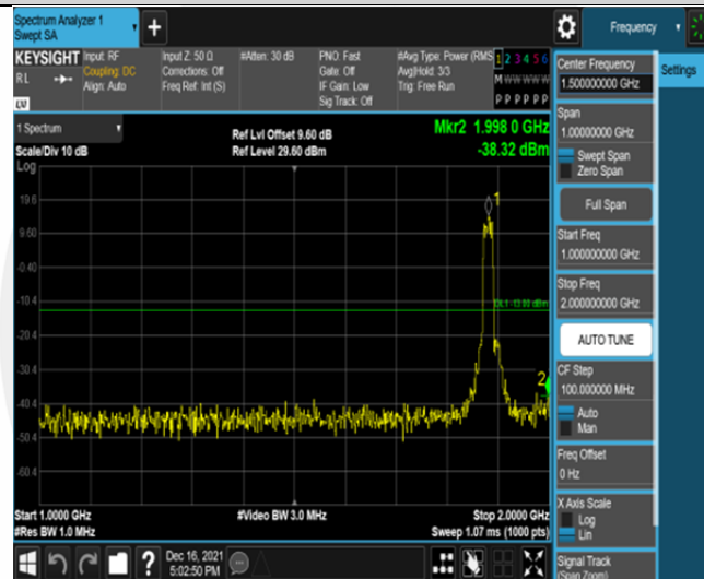
Band2-20MHz-16QAM-18900-100RB#0-Range2:1000~2000MHz
