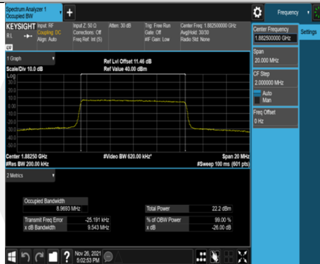
Band25-10MHz-16QAM-26365-50RB#0
