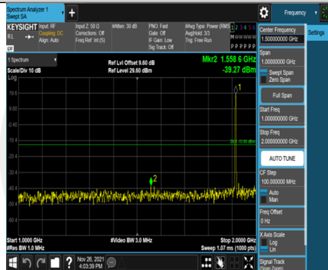
Band25-1.4MHz-QPSK-26683-6RB#0-Range2:1000~2000MHz
