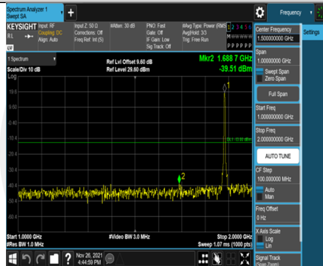
Band25-5MHz-QPSK-26365-25RB#0-Range2:1000~2000MHz
