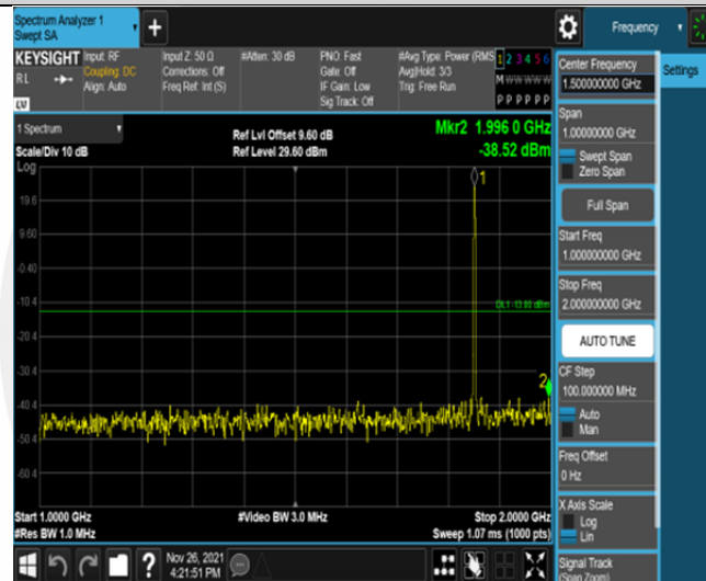
Band25-3MHz-QPSK-26055-1RB#0-Range2:1000~2000MHz
