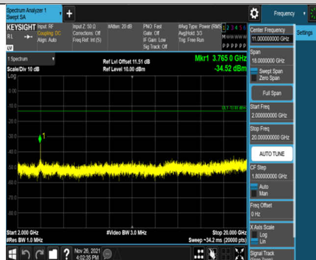
Band25-1.4MHz-QPSK-26365-6RB#0-Range3:2000~20000MHz
