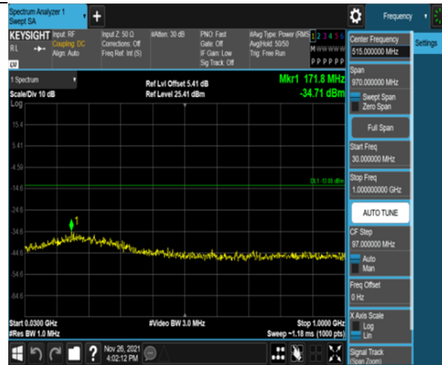
Band25-1.4MHz-QPSK-26365-6RB#0-Range1:30~1000MHz
