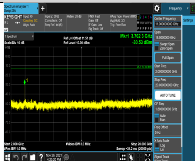
Band25-3MHz-QPSK-26365-1RB#0-Range3:2000~20000MHz
