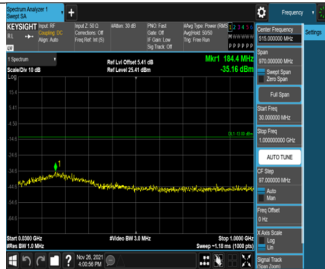
Band25-1.4MHz-QPSK-26047-6RB#0-Range1:30~1000MHz
