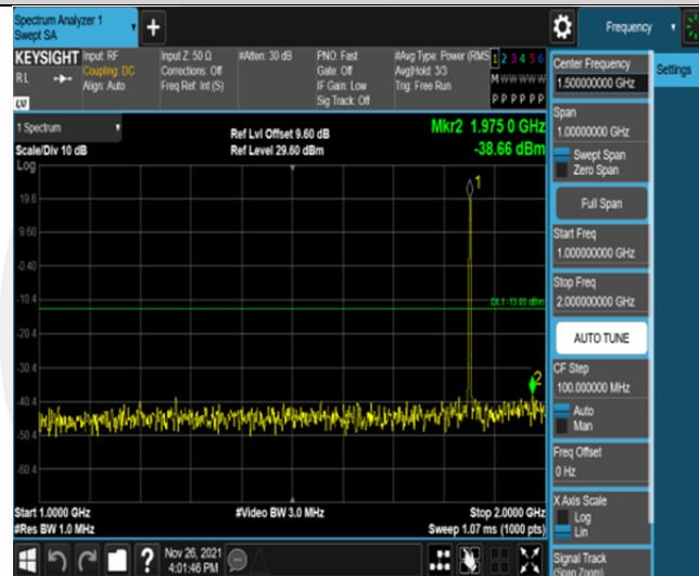
Band25-1.4MHz-16QAM-26047-6RB#0-Range2:1000~2000MHz
