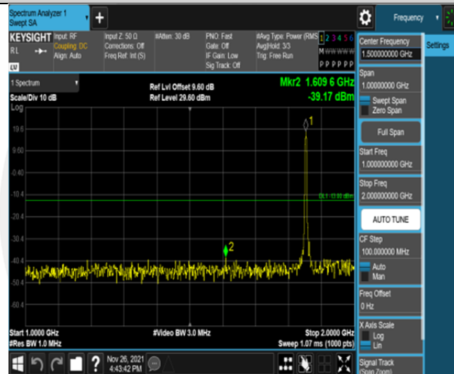
Band25-5MHz-QPSK-26065-25RB#0-Range2:1000~2000MHz
