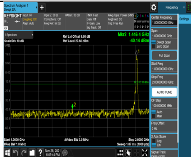
Band25-10MHz-QPSK-26640-50RB#0-Range2:1000~2000MHz
