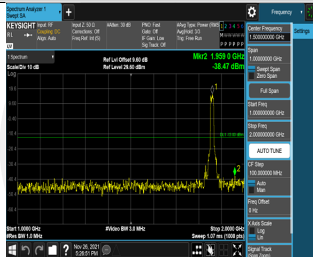
Band25-15MHz-QPSK-26115-75RB#0-Range2:1000~2000MHz
