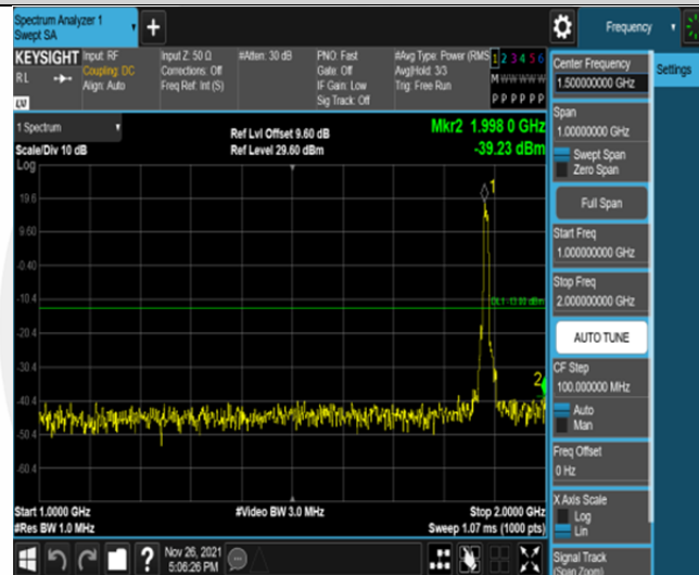
Band25-10MHz-QPSK-26365-50RB#0-Range2:1000~2000MHz
