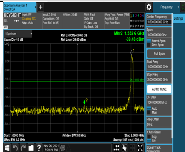
Band25-15MHz-QPSK-26615-75RB#0-Range2:1000~2000MHz
