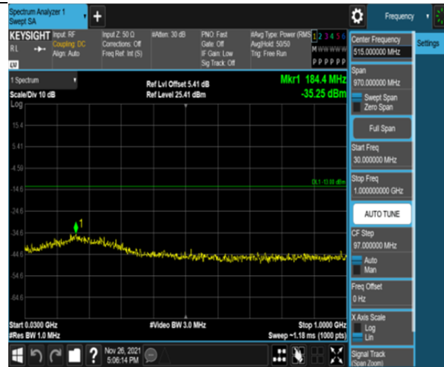
Band25-10MHz-QPSK-26365-50RB#0-Range1:30~1000MHz
