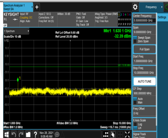
Band26-1.4MHz-QPSK-26697-6RB#0-Range2:1000~10000MHz
