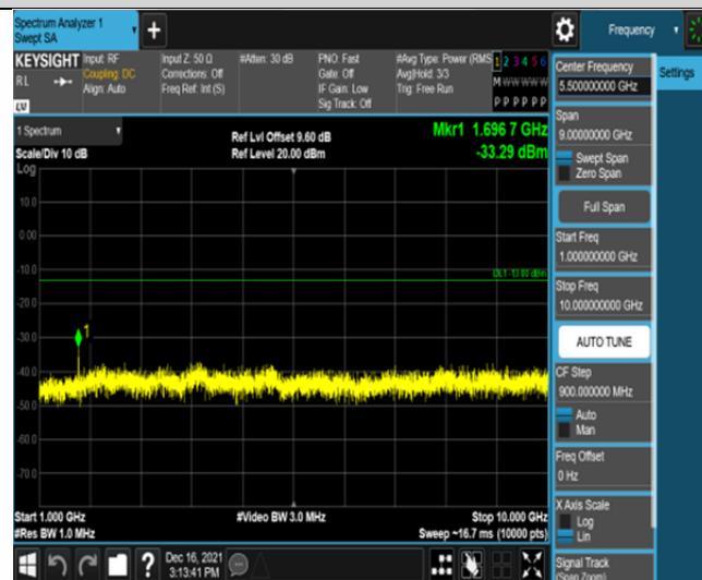
Band26-3MHz-QPSK-27025-15RB#0-Range2:1000~10000MHz
