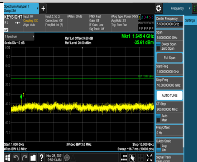
Band26-5MHz-QPSK-26765-25RB#0-Range2:1000~10000MHz
