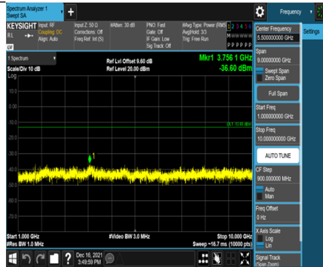
Band26-10MHz-QPSK-26840-50RB#0-Range2:1000~10000MHz
