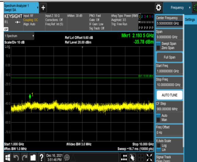
Band26-10MHz-QPSK-26990-50RB#0-Range2:1000~10000MHz
