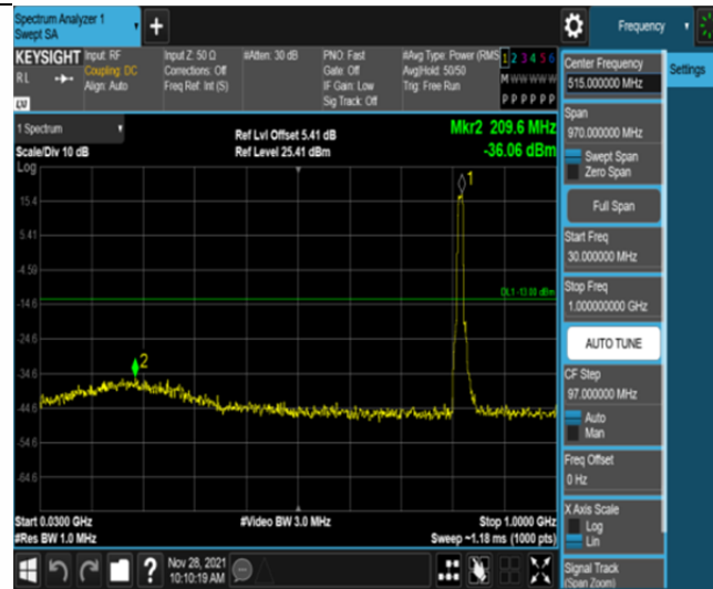
Band26-10MHz-QPSK-26740-50RB#0-Range1:30~1000MHz
