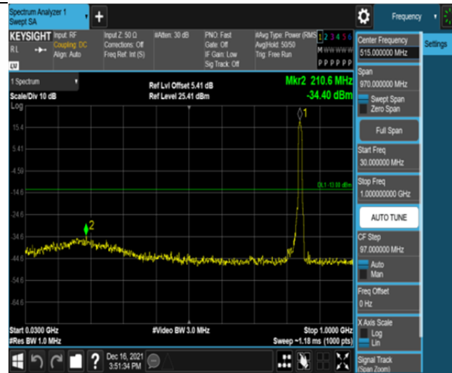
Band26-10MHz-QPSK-26990-50RB#0-Range1:30~1000MHz
