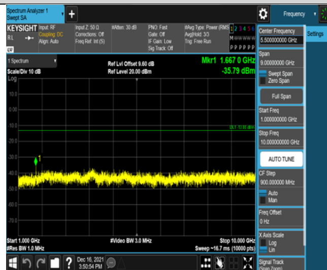
Band26-10MHz-QPSK-26915-50RB#0-Range2:1000~10000MHz
