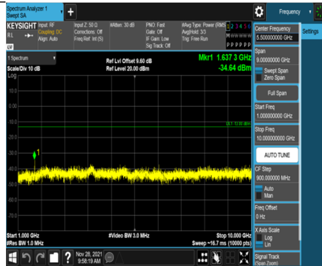
Band26-5MHz-QPSK-26740-25RB#0-Range2:1000~10000MHz
