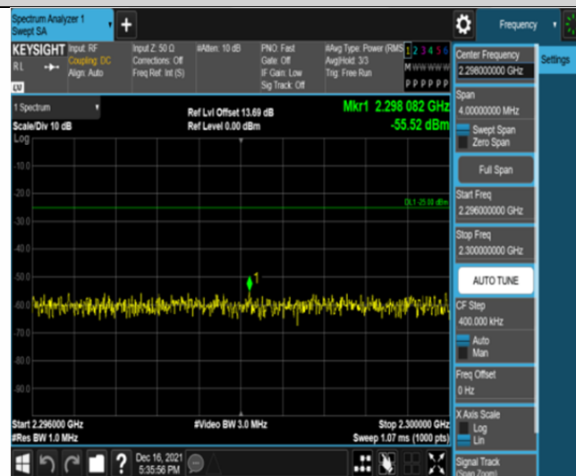
Band30-5MHz-QPSK-27710-25RB#0-Range5:2296~2300MHz
