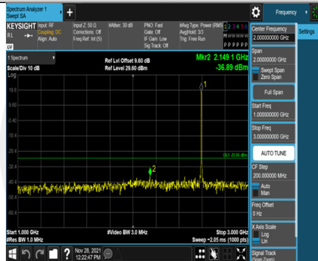
Band41-5MHz-QPSK-40620-25RB#0-Range2:1000~3000MHz
