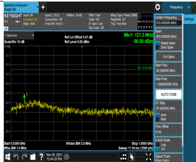
Band41-10MHz-QPSK-41540-50RB#0-Range1:30~1000MHz
