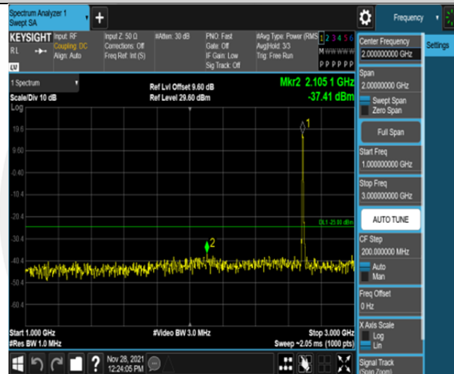
Band41-5MHz-QPSK-41565-25RB#0-Range2:1000~3000MHz
