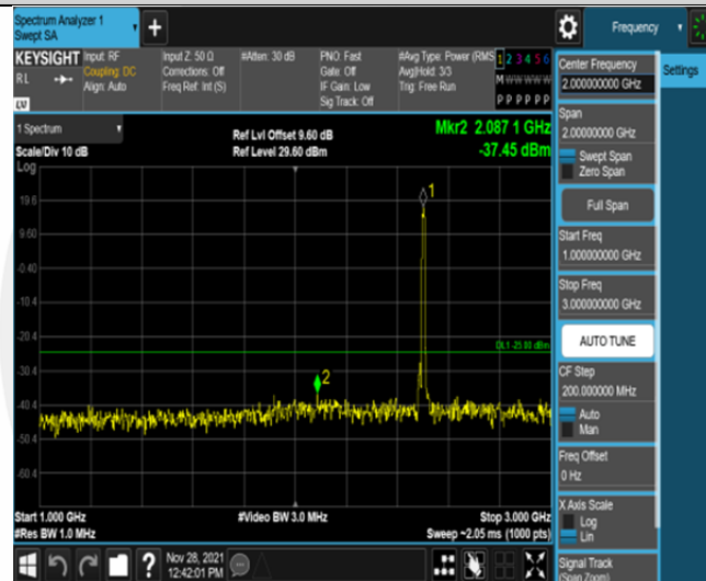
Band41-10MHz-QPSK-39700-50RB#0-Range2:1000~3000MHz
