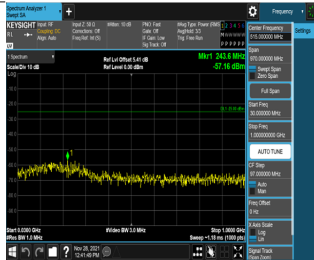
Band41-10MHz-QPSK-39700-50RB#0-Range1:30~1000MHz
