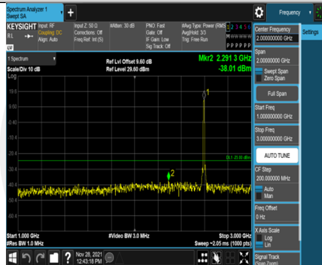
Band41-10MHz-QPSK-40620-50RB#0-Range2:1000~3000MHz
