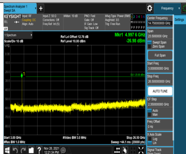
Band41-5MHz-QPSK-39675-25RB#0-Range3:3000~26500MHz
