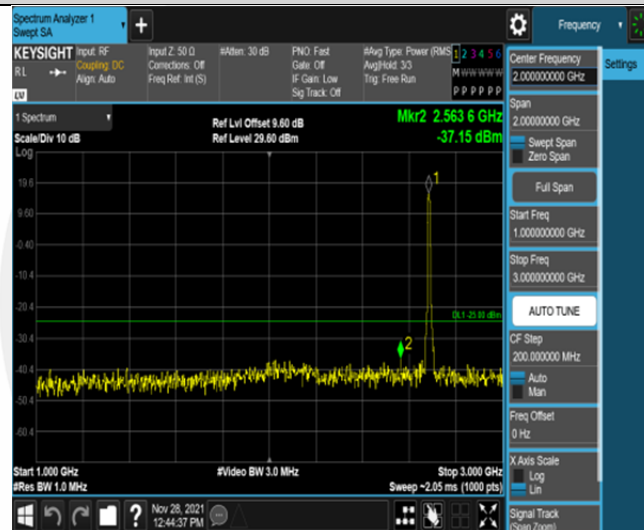
Band41-10MHz-QPSK-41540-50RB#0-Range2:1000~3000MHz
