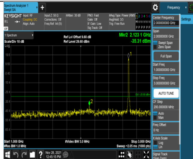
Band41-10MHz-16QAM-41540-50RB#0-Range2:1000~3000MHz
