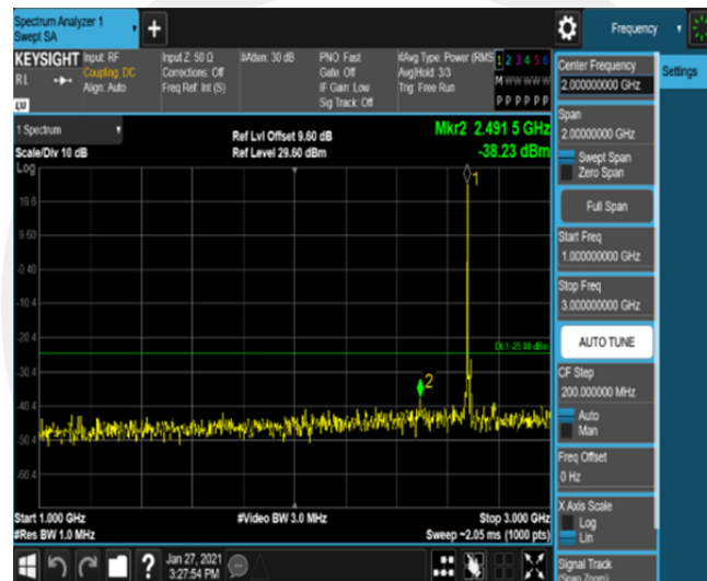
Band41-20MHz-QPSK-39750-100RB#0-Range2:1000~3000MHz
