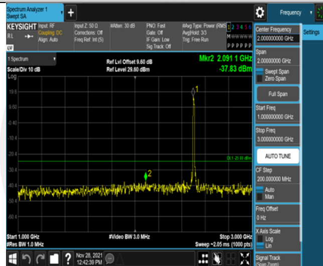
Band41-10MHz-16QAM-39700-50RB#0-Range2:1000~3000MHz
