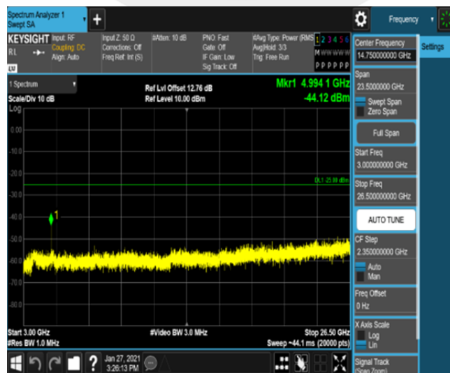
Band41-10MHz-16QAM-41540-50RB#0-Range3:3000~26500MHz
