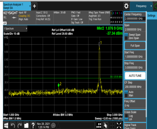
Band41-20MHz-QPSK-40620-100RB#0-Range2:1000~3000MHz
