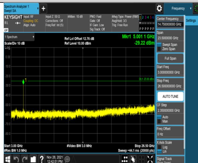
Band41-10MHz-16QAM-39700-50RB#0-Range3:3000~26500MHz
