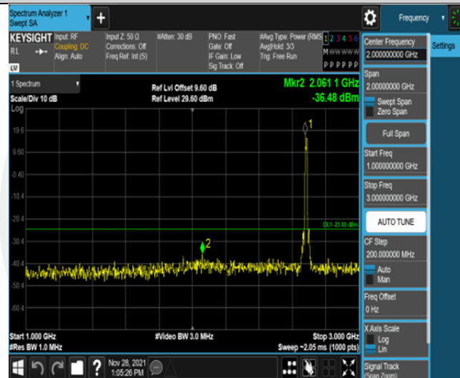
Band41-15MHz-QPSK-41515-75RB#0-Range2:1000~3000MHz
