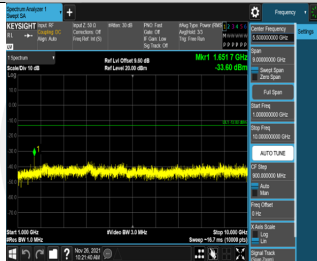
Band5-3MHz-QPSK-20415-15RB#0-Range2:1000~10000MHz
