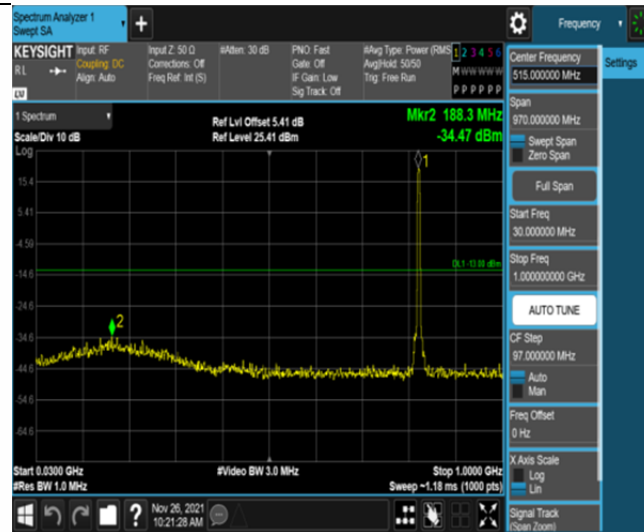
Band5-3MHz-QPSK-20415-15RB#0-Range1:30~1000MHz
