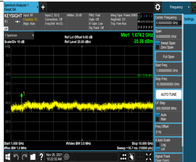
Band5-3MHz-QPSK-20525-15RB#0-Range2:1000~10000MHz
