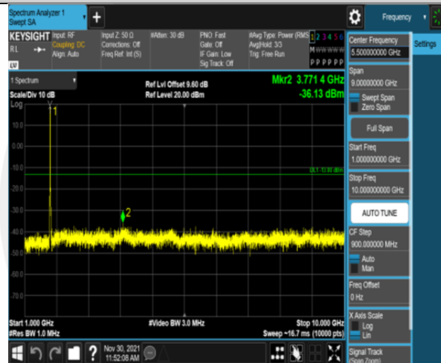
Band66-10MHz-QPSK-132022-50RB#0-Range2:1000~10000MHz
