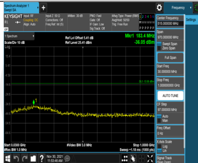
Band66-10MHz-QPSK-132622-50RB#0-Range1:30~1000MHz
