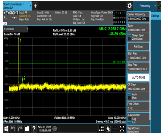
Band66-10MHz-QPSK-132322-50RB#0-Range2:1000~10000MHz
