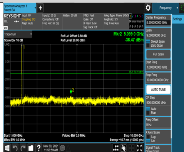
Band66-10MHz-QPSK-132622-50RB#0-Range2:1000~10000MHz
