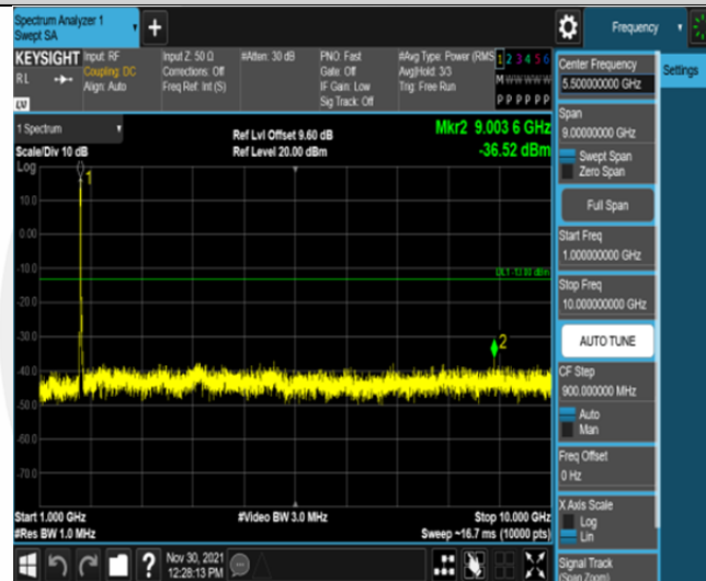
Band66-20MHz-QPSK-132072-100RB#0-Range2:1000~10000MHz
