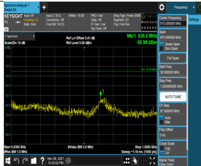
Band7-10MHz-QPSK-21400-50RB#0-Range1:30~1000MHz
