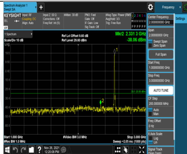
Band7-5MHz-QPSK-21100-25RB#0-Range2:1000~3000MHz
