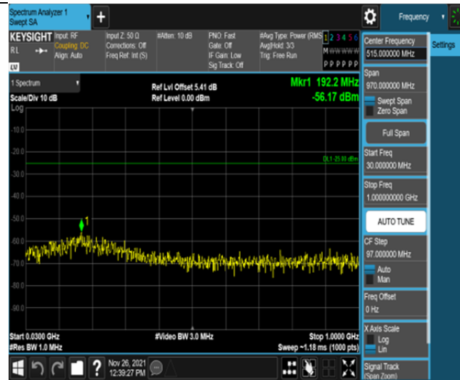
Band7-10MHz-QPSK-20800-50RB#0-Range1:30~1000MHz
