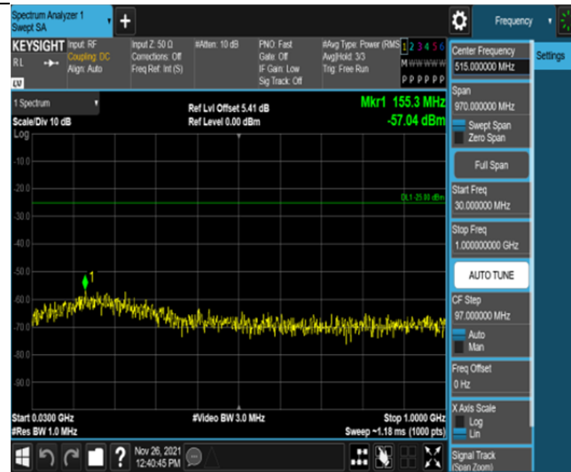
Band7-10MHz-QPSK-21100-50RB#0-Range1:30~1000MHz
