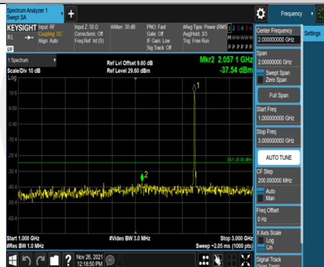
Band7-5MHz-QPSK-20775-25RB#0-Range2:1000~3000MHz
