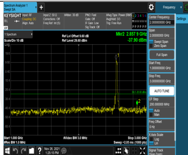
Band7-20MHz-16QAM-21350-100RB#0-Range2:1000~3000MHz
