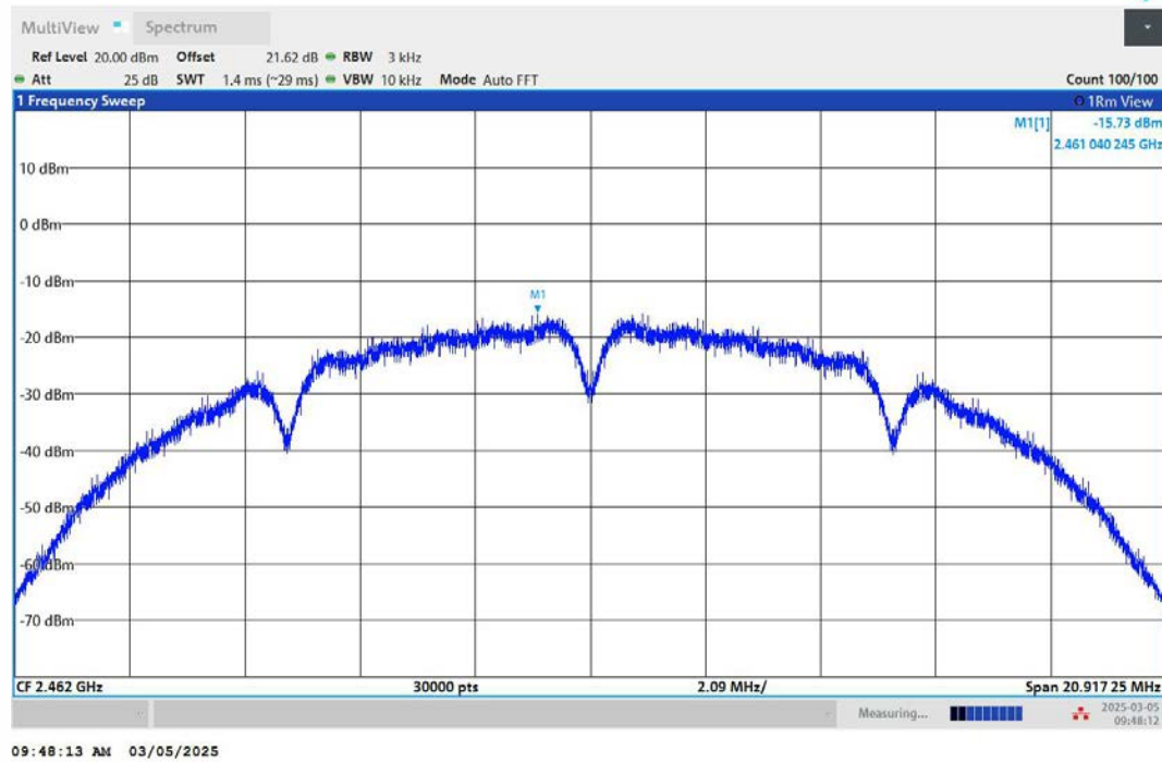
11B-Ant2-2462-PASS
